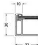
Keret hosszú oldal keresztmetszete
